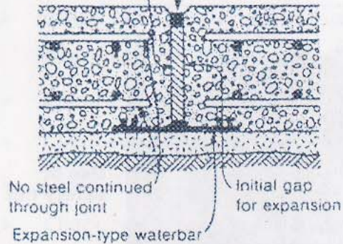
(d) Expansion joint in reservoir wall
