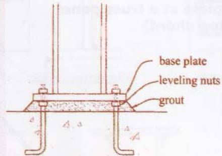
Leveling nuts
